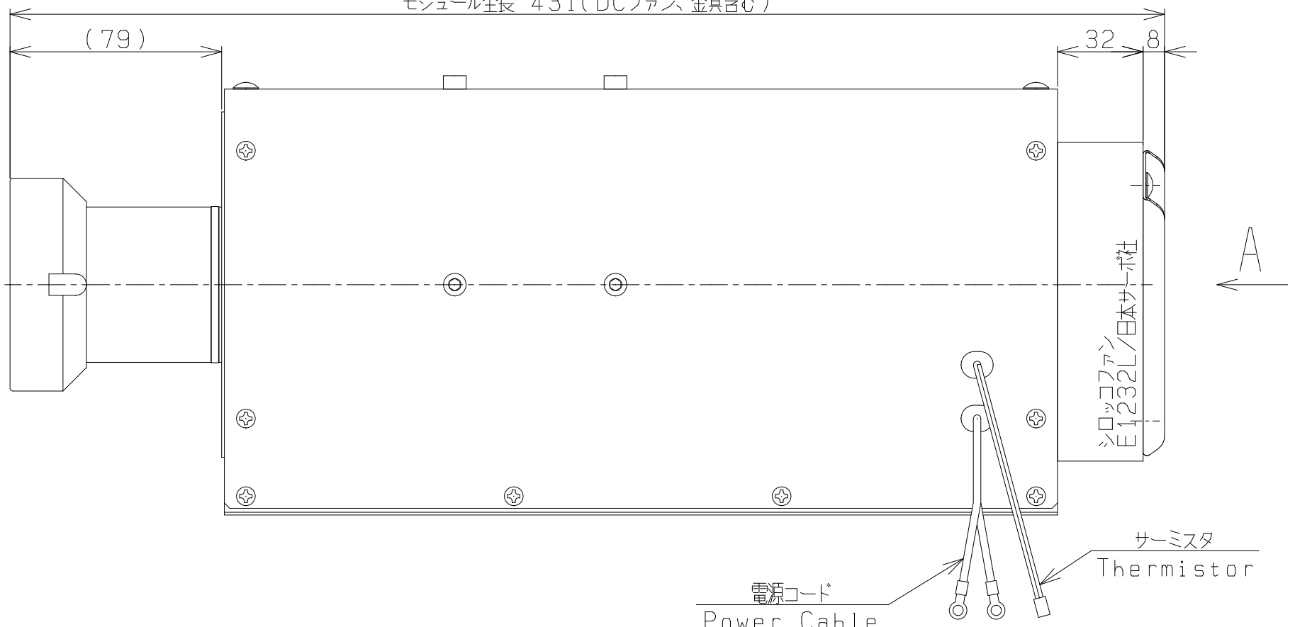
Module Size モジュール全長 431 (DCファン、金具含む)
