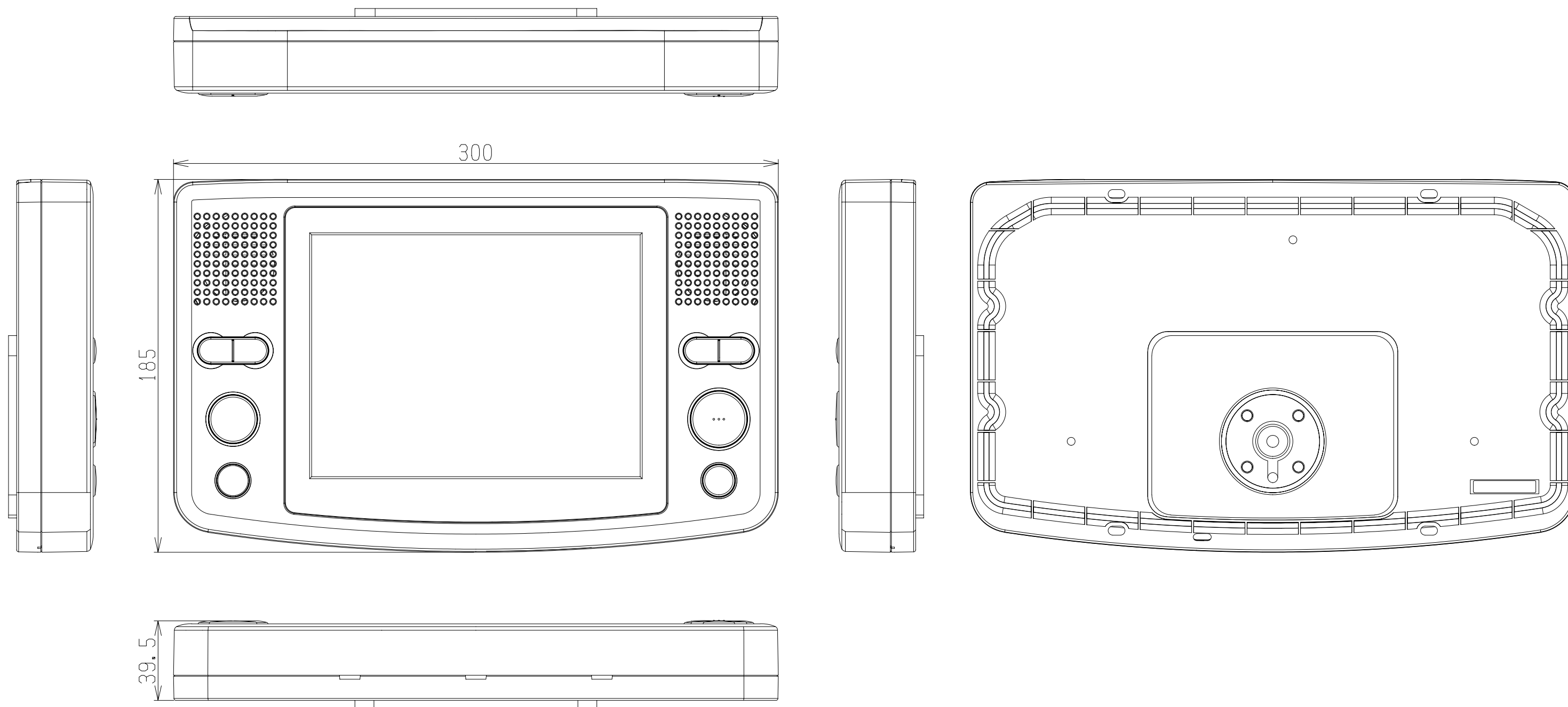
VB-J821 8型浴室テレビ外形寸法図
