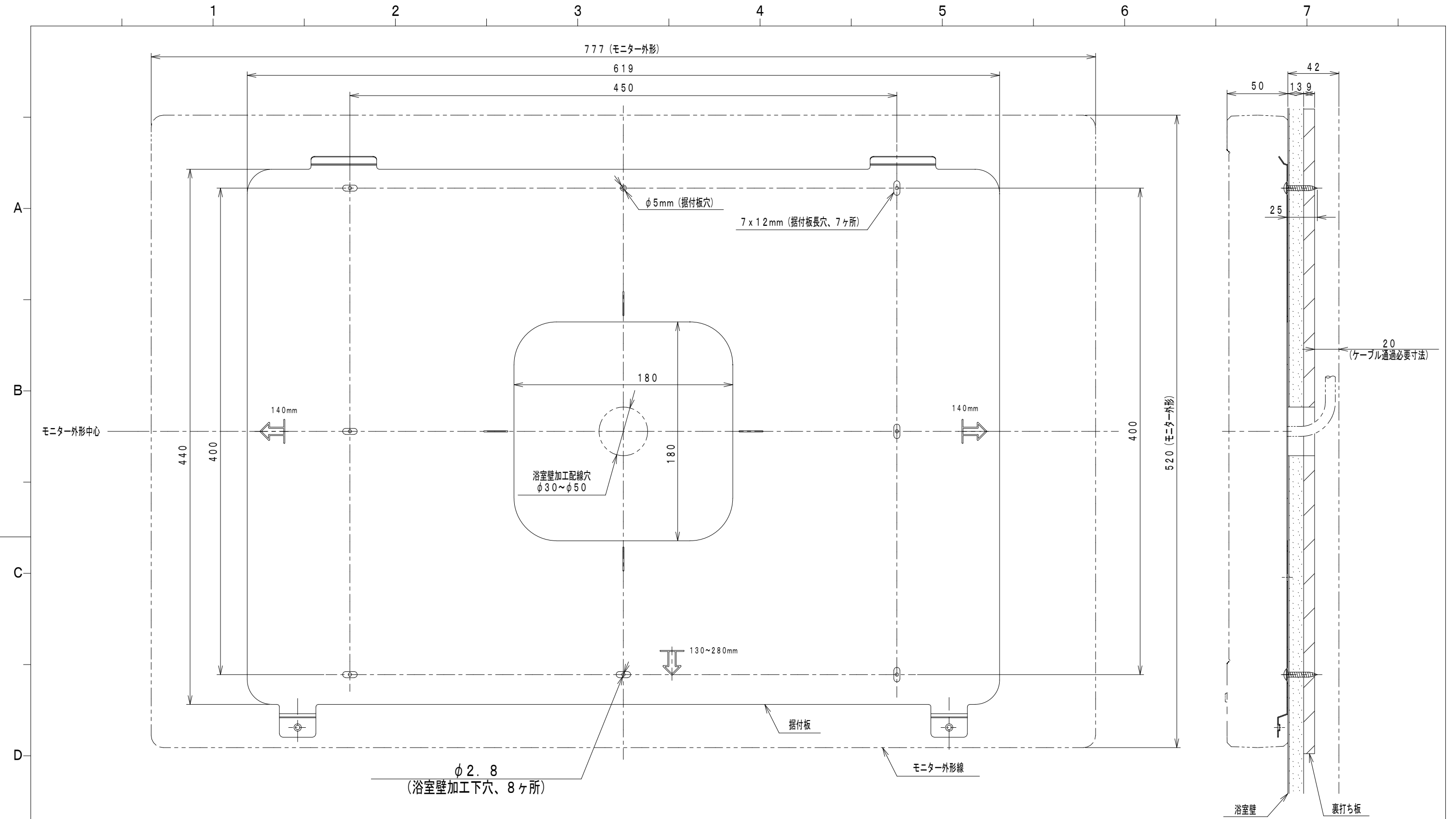
浴室壁加工穴寸法図
