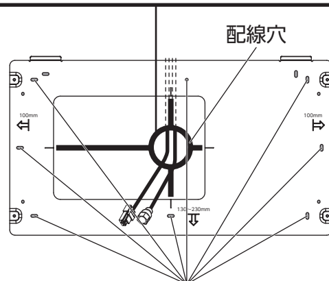
壁据付板取付けに使用する穴の位置
