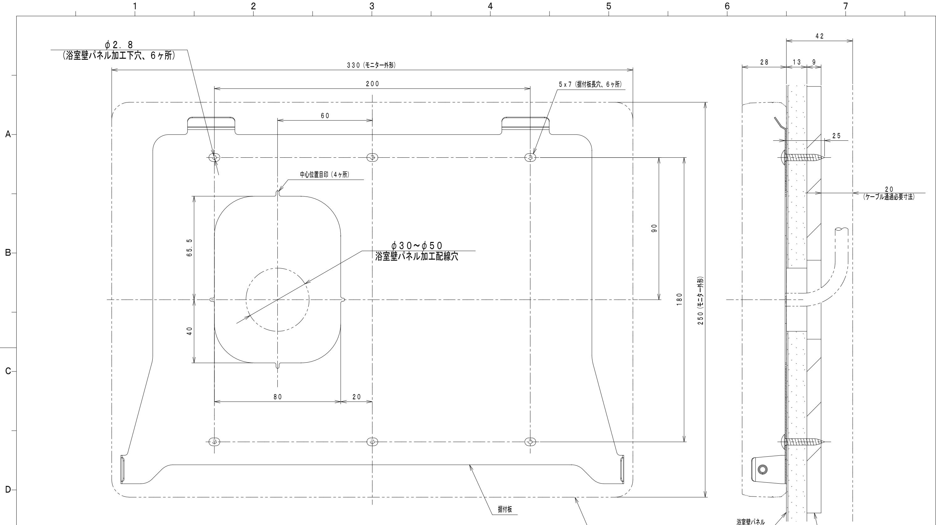
浴室壁パネル加工穴寸法図
